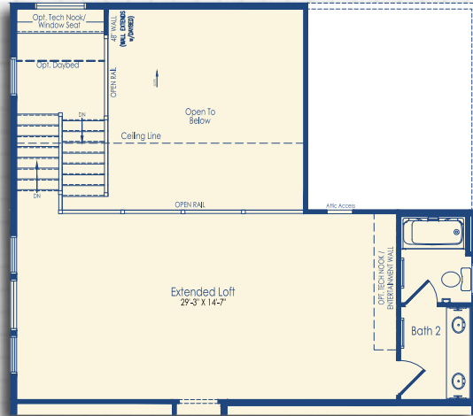
Optional Extended Loft
