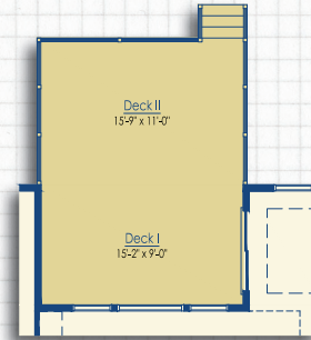
Optional Deck I & Optional Deck II
