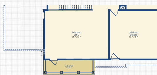
Optional Extended Loft 2 Elevation C
