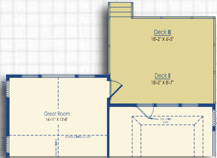
Optional Deck II
