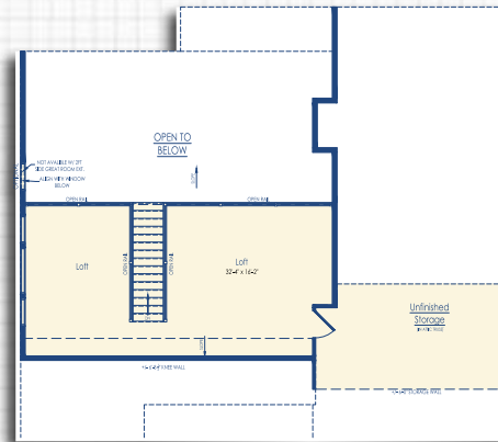
Optional Loft Elevation A/B
