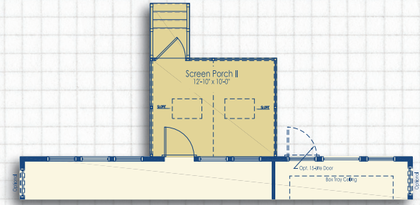
Optional Screen Porch I
