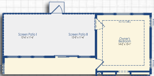
Optional Screen Patio I & II
