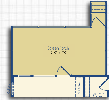
Optional Screen Porch I
