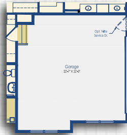
Optional Side Load Schell Style C
