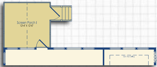
Optional Screen Porch I
