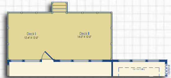
Optional Optional Deck I and Deck II
