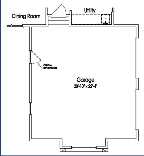
OPTIONAL SIDE LOAD GARAGE
