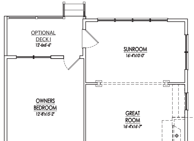
OPTIONAL SUNROOM W/ OPTIONAL DECK I
